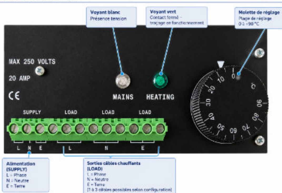
Vue intérieure du ELTH-A6
